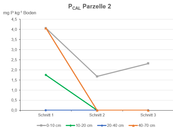
Abbildung 31: P CAL Parzelle 2, eigene Darstellung
