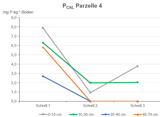
Abbildung 35: P CAL Parzelle 4, eigene Darstellung
