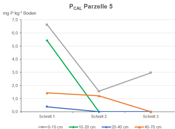
Abbildung 37: P CAL Parzelle 5, eigene Darstellung
