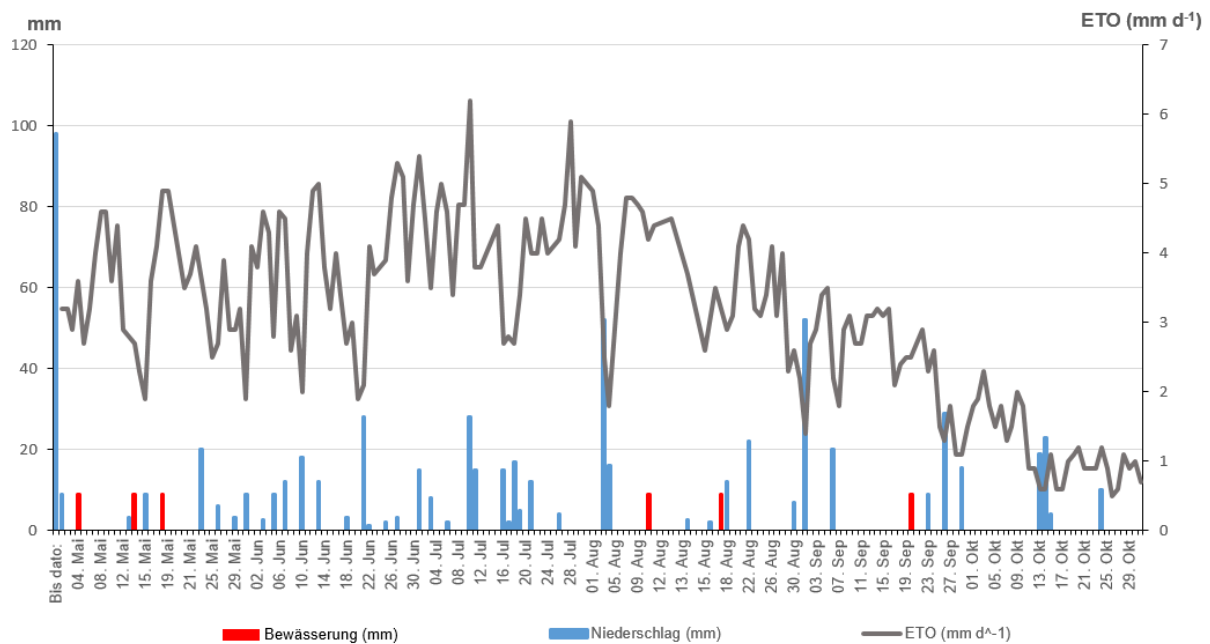
Abbildung 26: Potenzielle tägliche Evapotranspiration, eigene Darstellung 4
