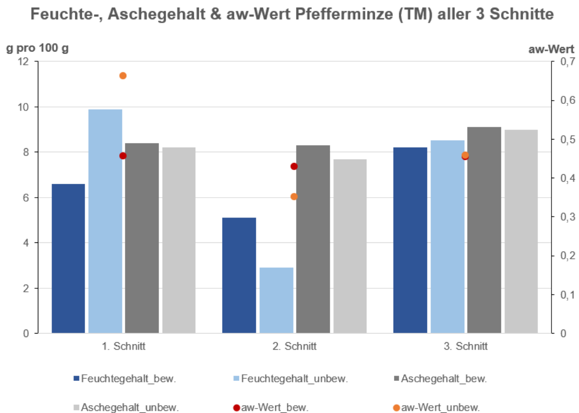
Abbildung 47: Feuchte-, Aschegehalt und aw-Wert aller drei Schnitte, eigene Darstellung
