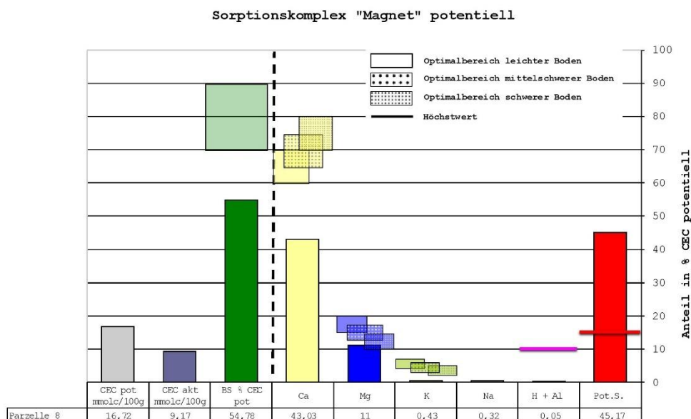
Abbildung: Zusammensetzung der potentiellen Austauscherkapazität (CEC pot)
