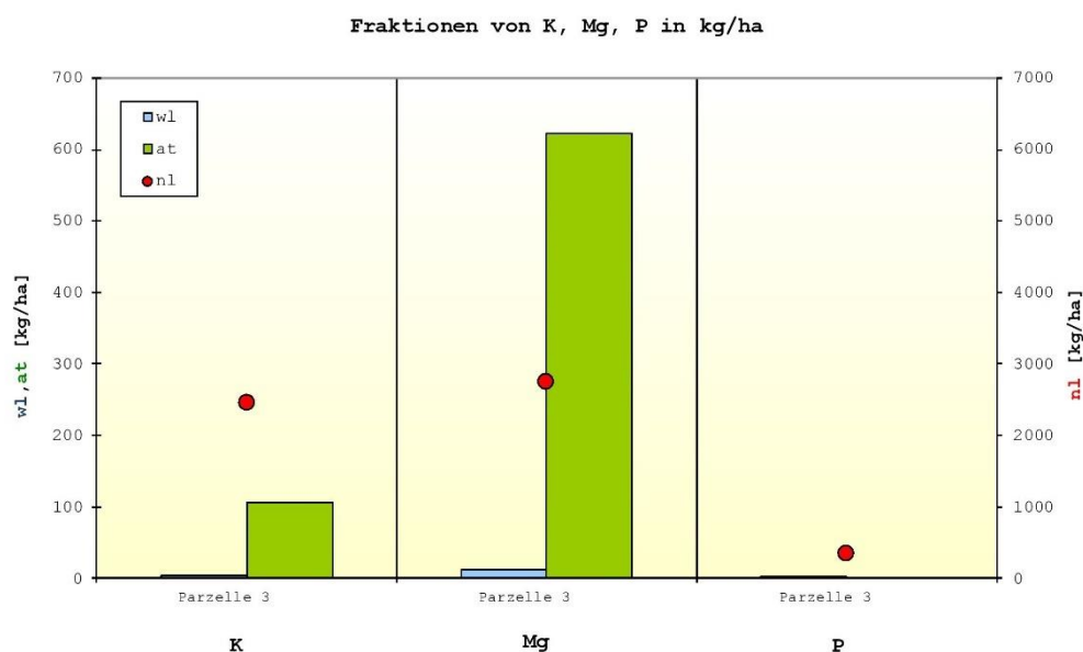
Abbildung: Fractionen der Nährstoffe K, Mg, P (wl=wasserlöslich, at=austauschbar, nl=nachlieferbar). Alle Gehalte sind Nettowerte (at ohne wl, nl ohne at und ohne wl)
