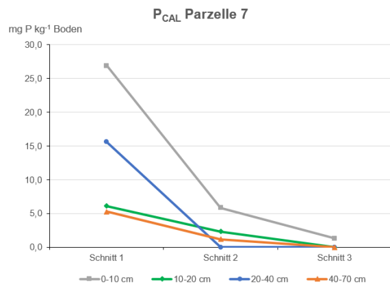
Abbildung 32: P CAL Parzelle 7, eigene Darstellung
