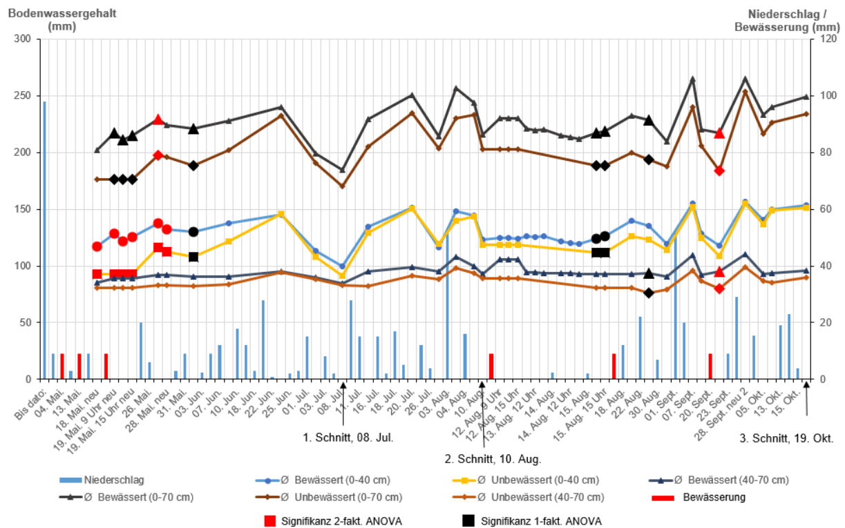
Abbildung 20: Volumetrischer Bodenwassergehalt, Varianzanalyse, eigene Darstellung 3
