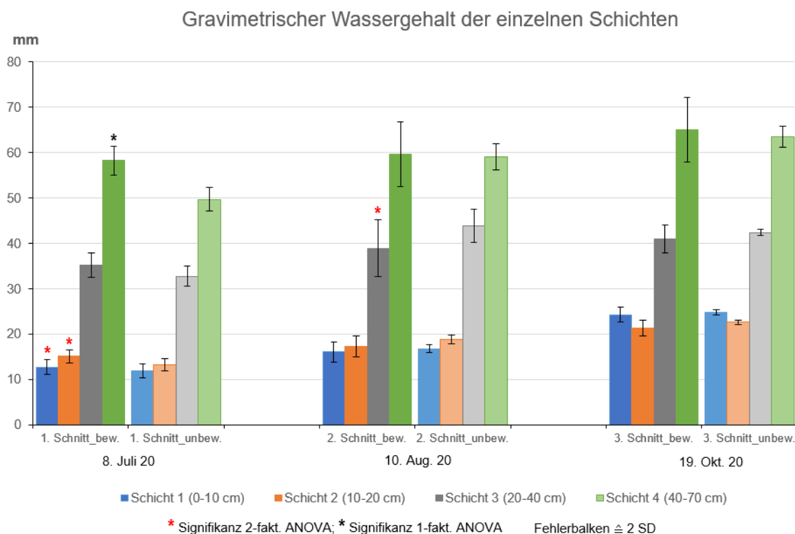
Abbildung 24: Varianzanalyse grav. WG der einzelnen Schichten, eigene Darstellung
