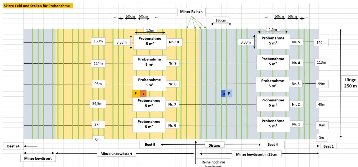
Abbildung 18: Profilstellen Wurzelbild, eigene Darstellung
