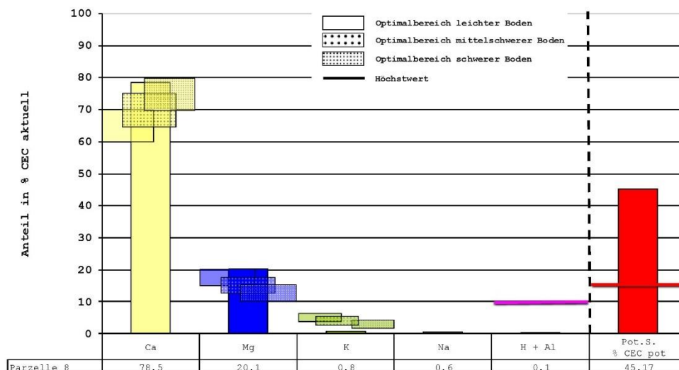
Abbildung: Zusammensetzung der aktuellen Austauschkapazität (CEC akt) sowie Anteil der potentiellen Säure (Pot. S.) am CEC pot
