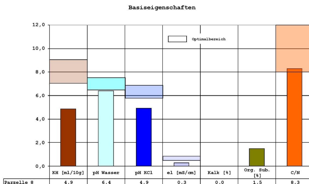
Abbildung: Basiseigenschaften des Bodens
