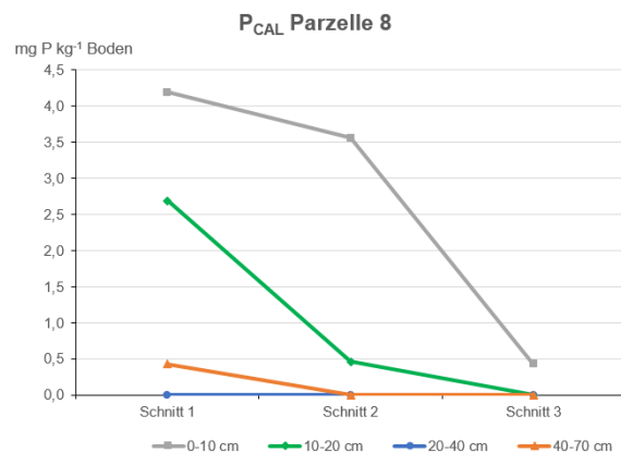
Abbildung 34: P CAL Parzelle 8, eigene Darstellung
