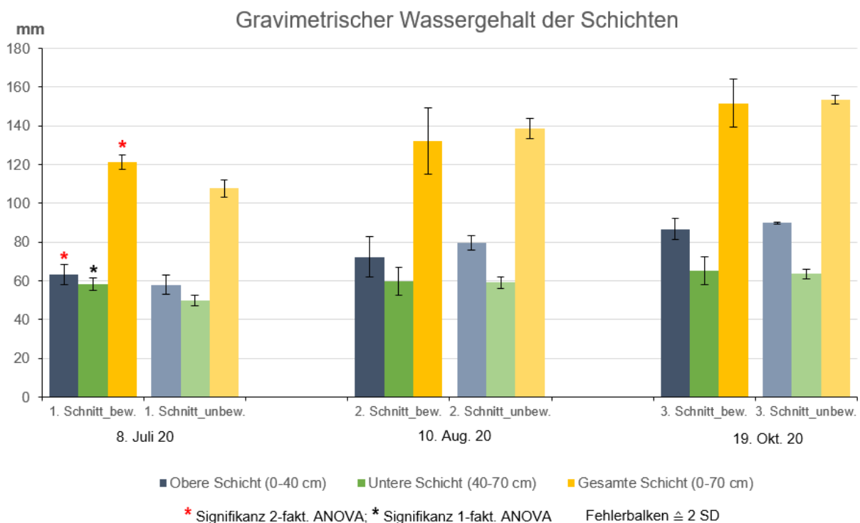
Abbildung 25: Varianzanalyse grav. WG der gesamten Schichten, eigene Darstellung
